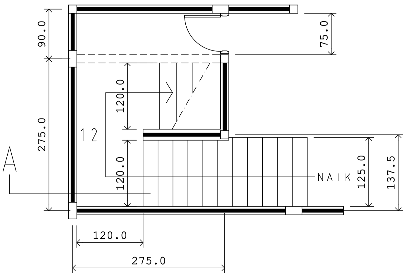
DENAH TANGGA NAIK
