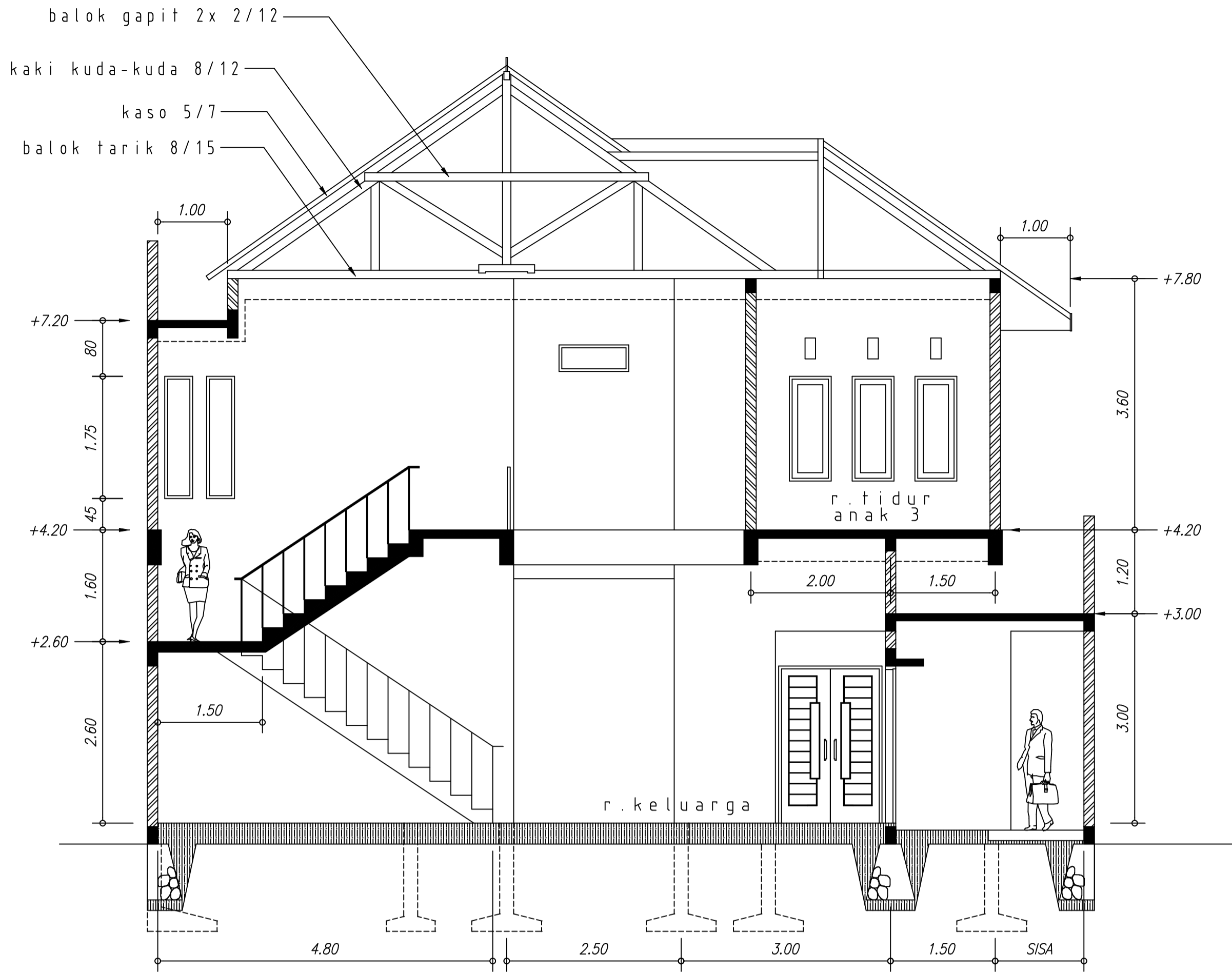
potongan B skala 1:100
